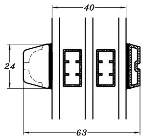
24 mm vandret energisprosse
