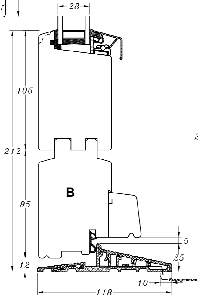
M/ alu.-bundtrin (standard)
