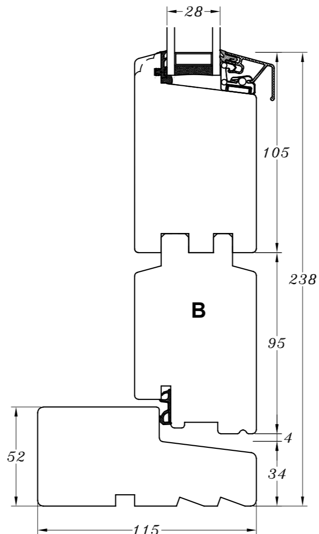
M/ træ-bundtrin
