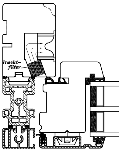
Klikventil på udadgående vindue med aftræk i fals
