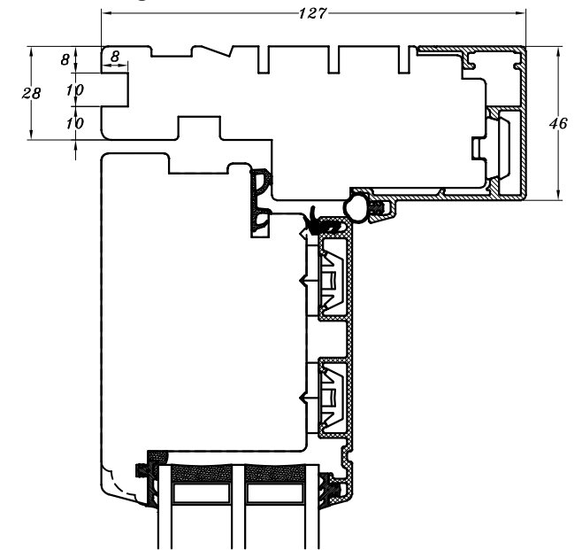
10 mm lysningsnot i side og top på indadgående dør
