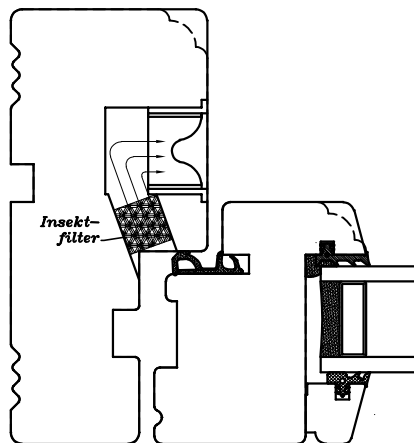
Klikventil på udadgående vindue med aftræk i fals
